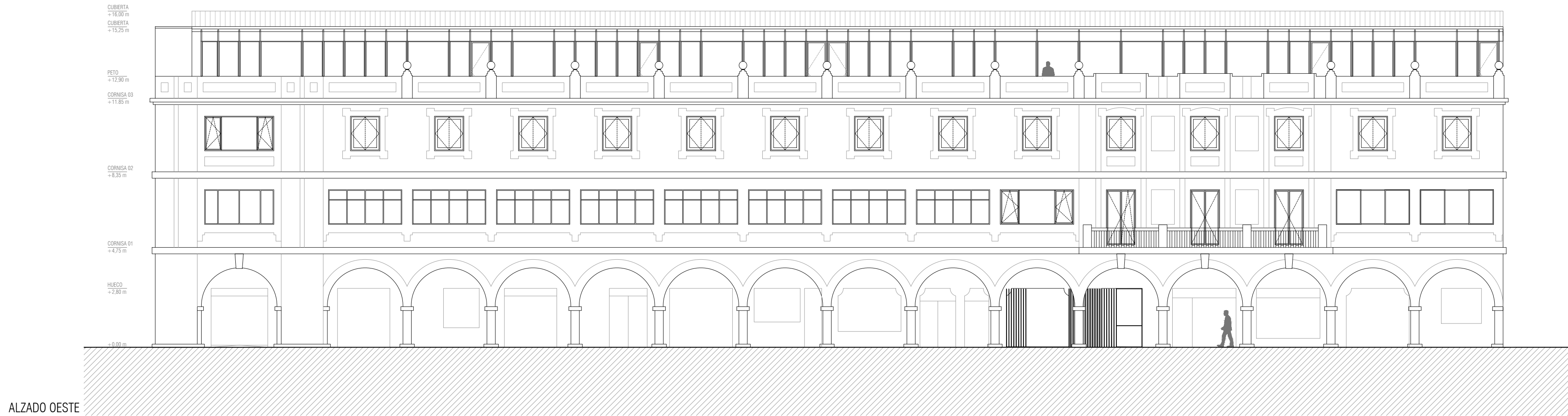
ALZADO OESTE
