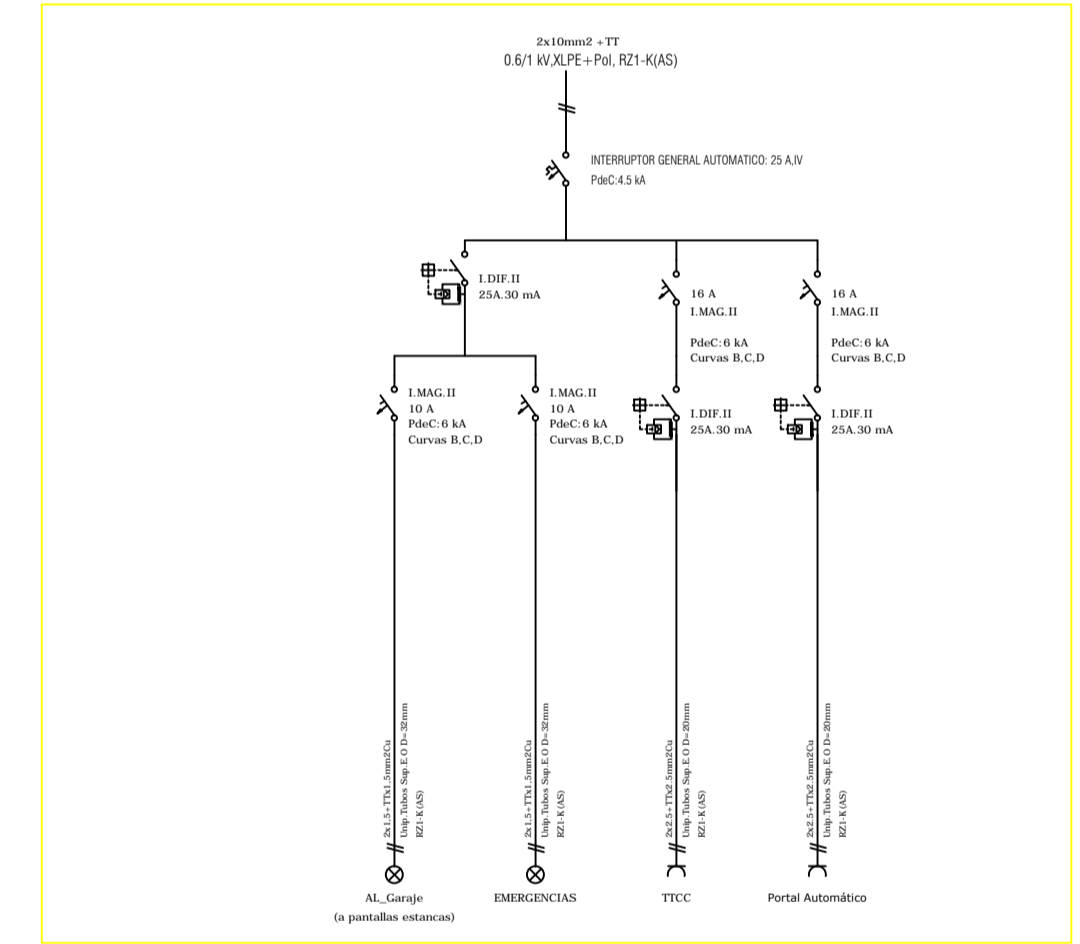
SURCUADRO DE PROTECCION GARAJES
