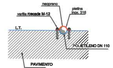
DETALLE B
