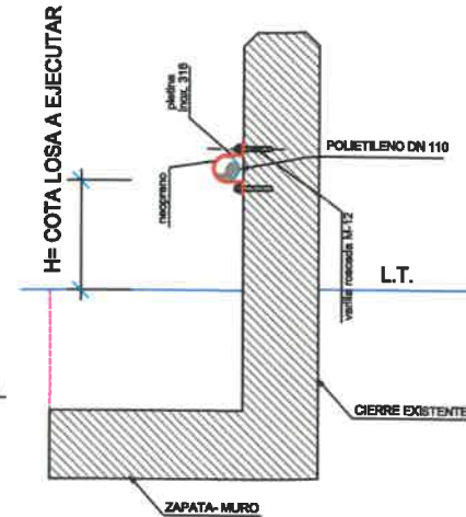
DETALLE A
