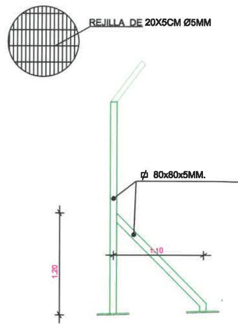
SECCIÓN A-A CERRAMIENTO
